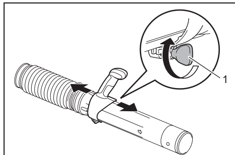
► 1. Clamp screw
